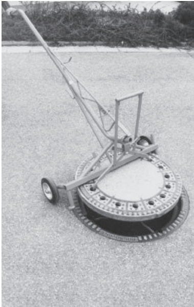
Schachtdeckel Hebewagen HR für runde Deckel
