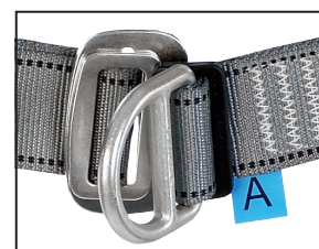
Steckverschluss mit Steigschutzöse (Brust), geschmiedeter Stahl
